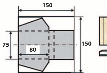
Рис. 2 Заготовки корпуса и накладки
